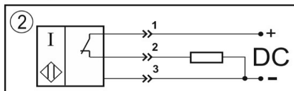
Нормально-замкнутый контакт
