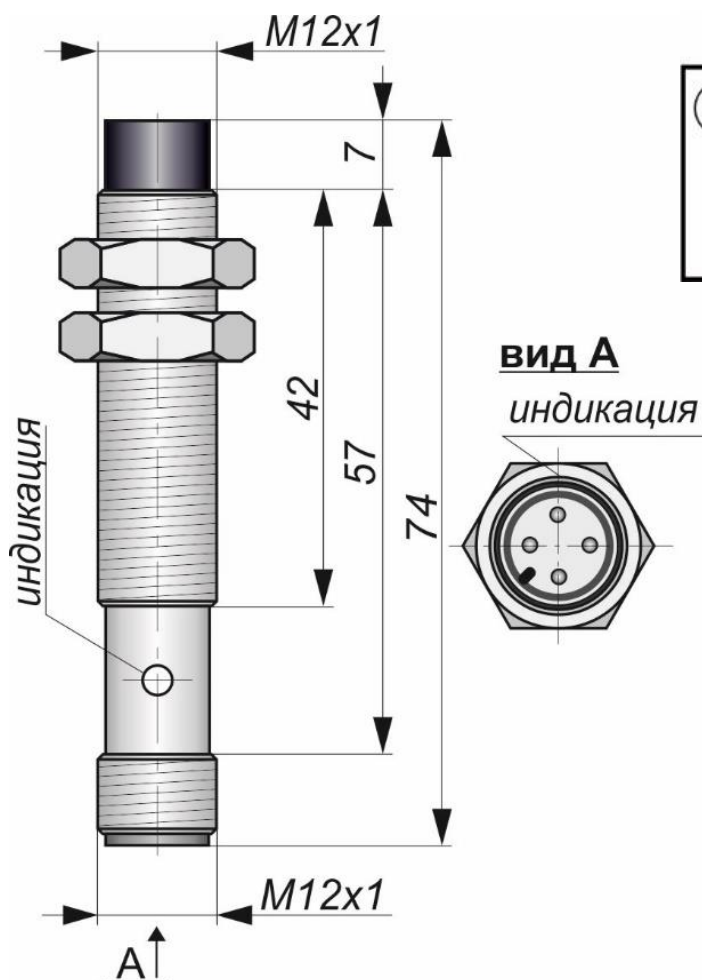
Габаритный чертеж
