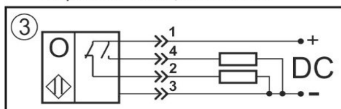
Цоколевка разъема
