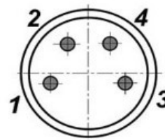
Цоколевка разъема
