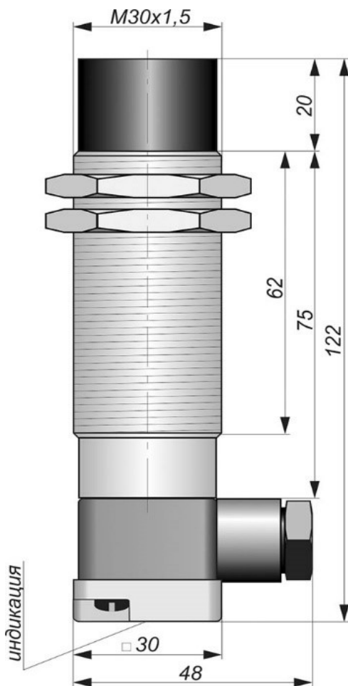
Габаритный чертеж
