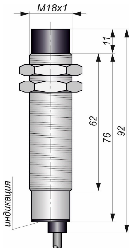
Габаритный чертеж
