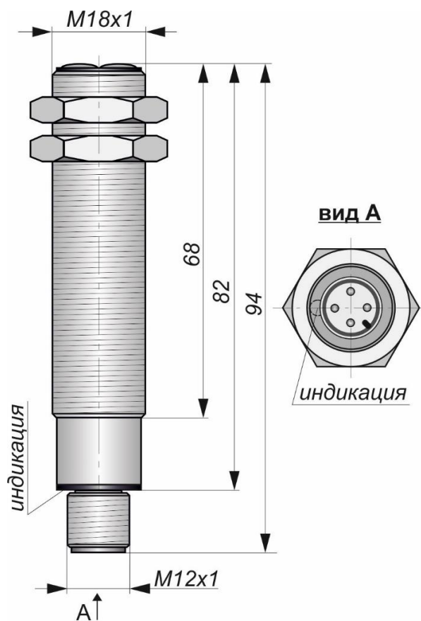
Габаритный чертеж
