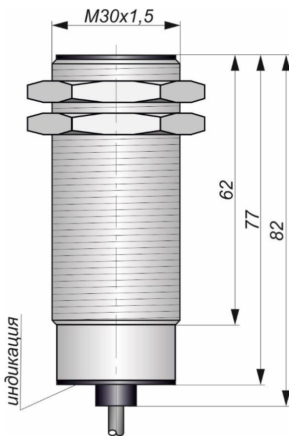
Габаритный чертеж
