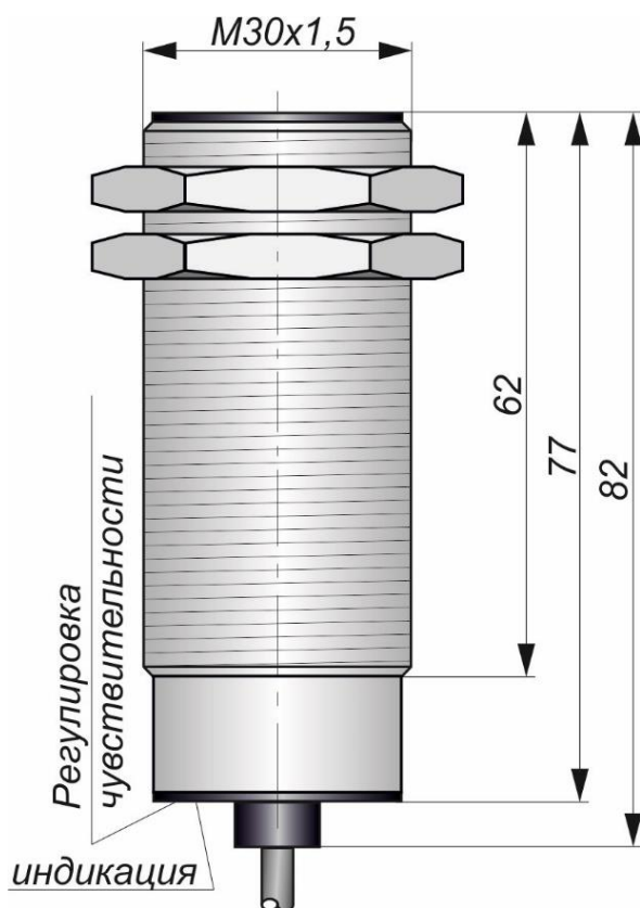
Габаритный чертеж
