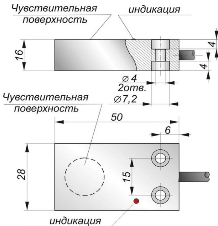
Габаритный чертеж
