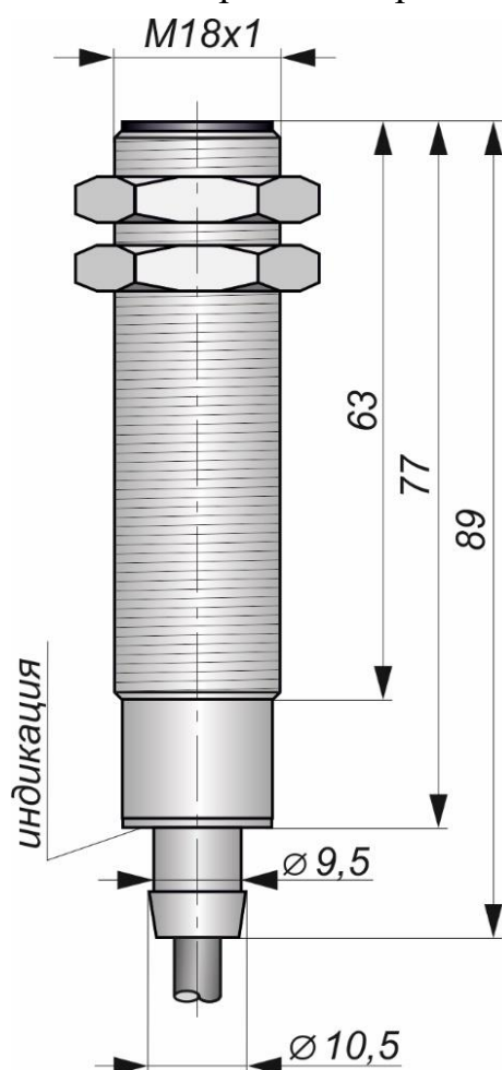
Габаритный чертеж
