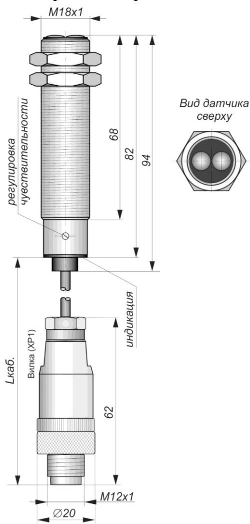
Габаритный чертеж
