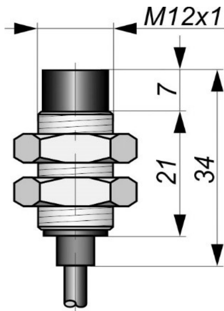
Габаритный чертеж
