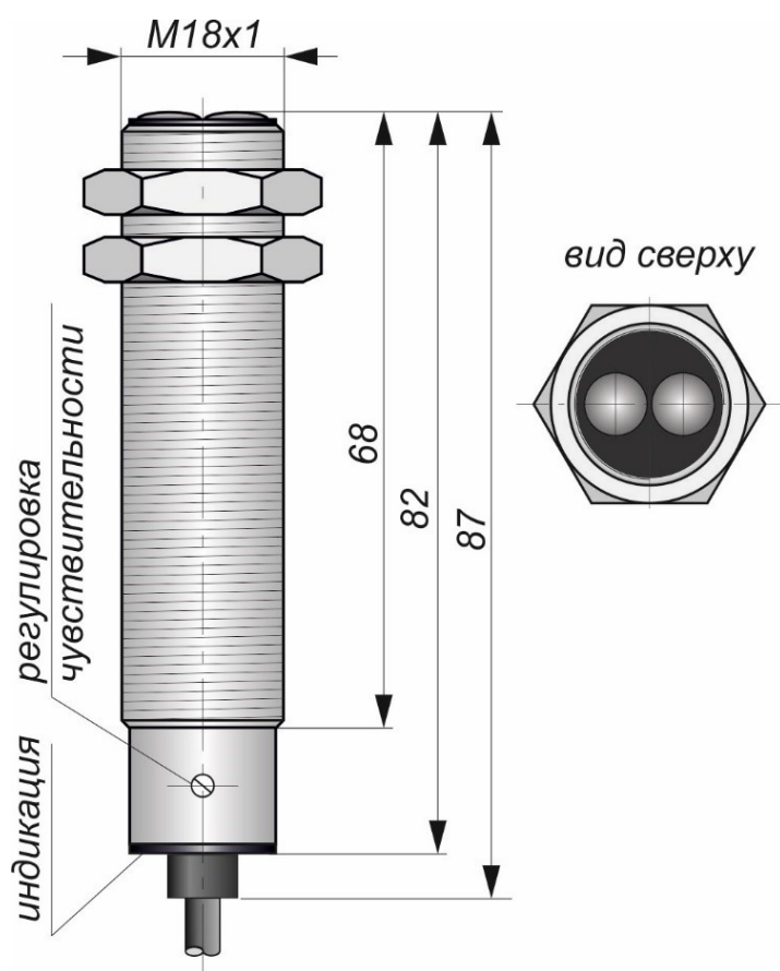
Габаритный чертеж
