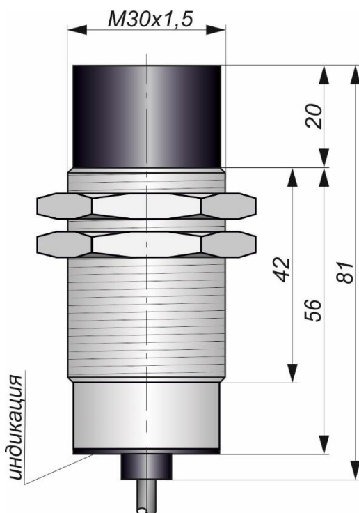
Габаритный чертеж
