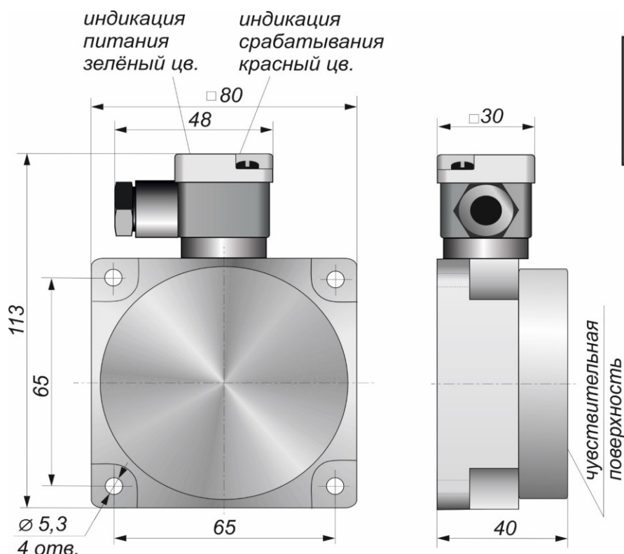
Габаритный чертеж
