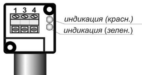
Цоколевка клеммной колодки
