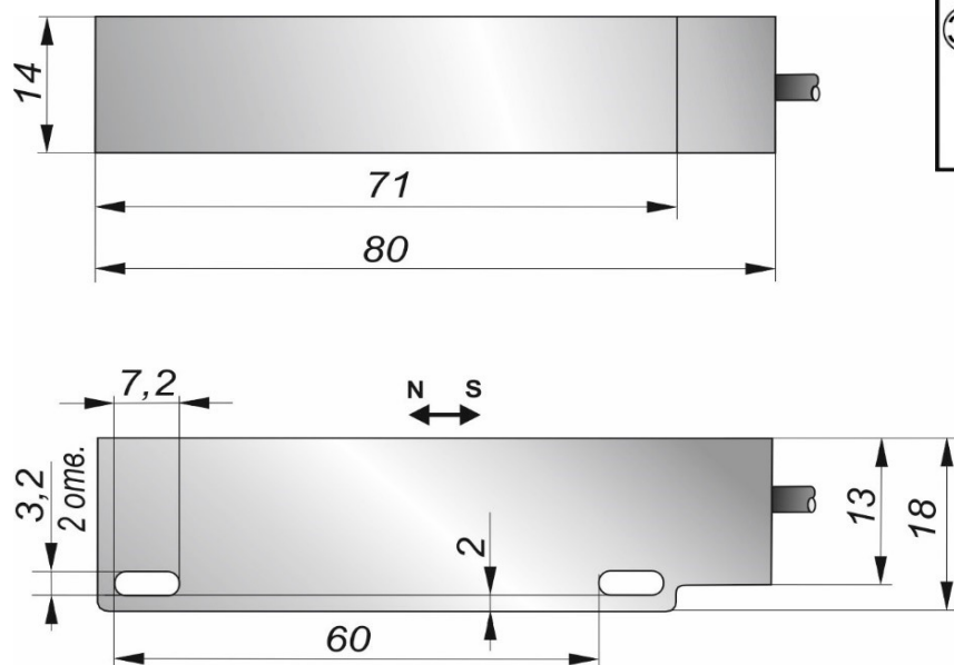
Габаритный чертеж
