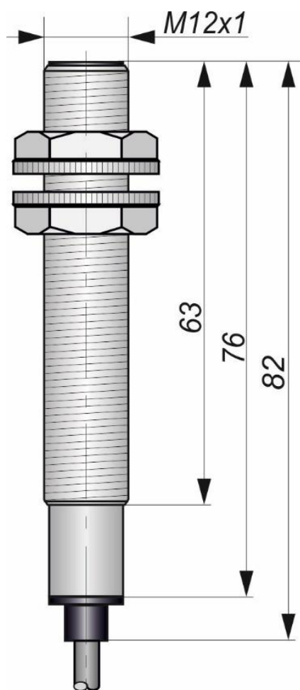
Габаритный чертеж
