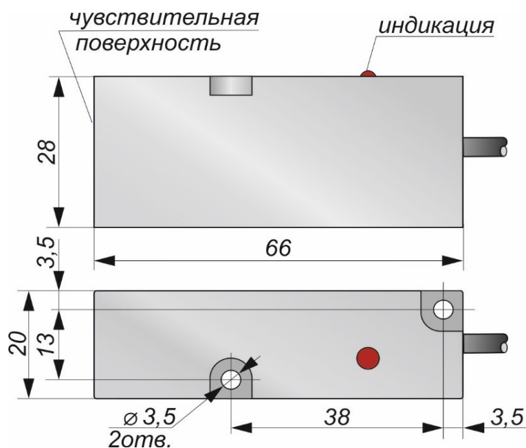
Габаритный чертеж
