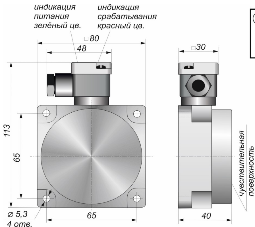
Габаритный чертеж
