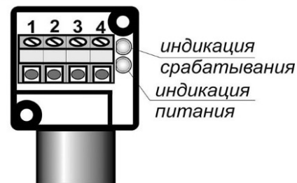
Цоколевка клеммной колодки
