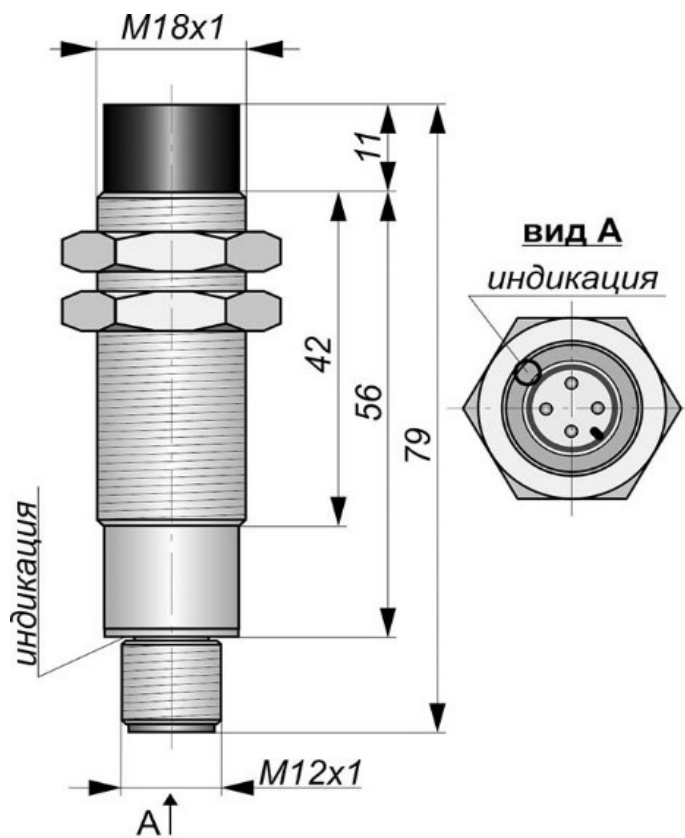
Габаритный чертеж
