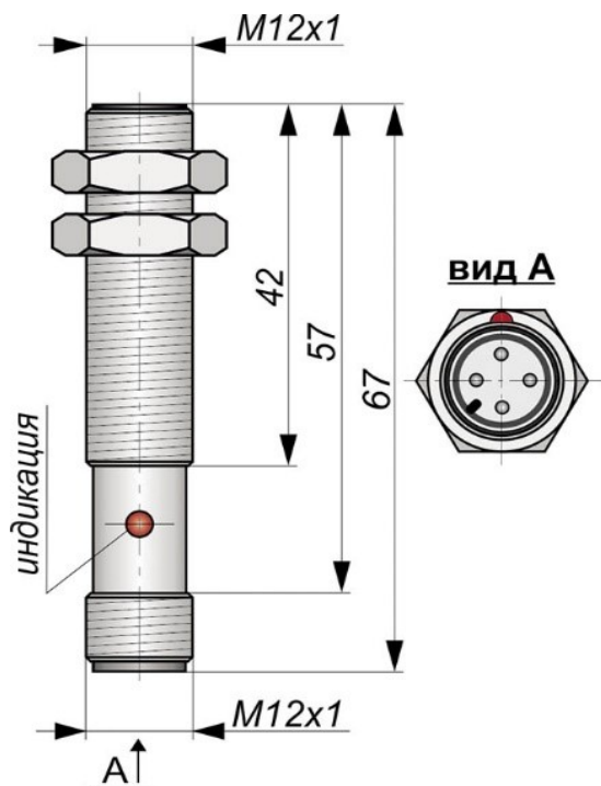
Габаритный чертеж
