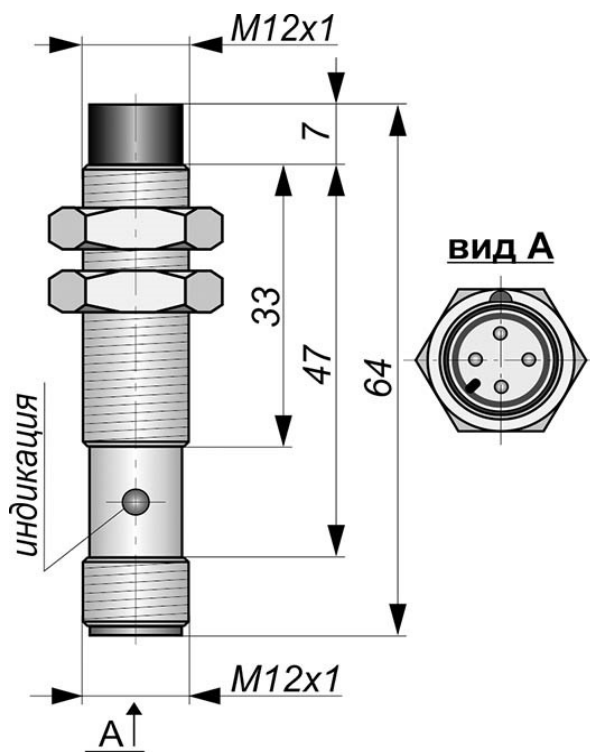
Габаритный чертеж
