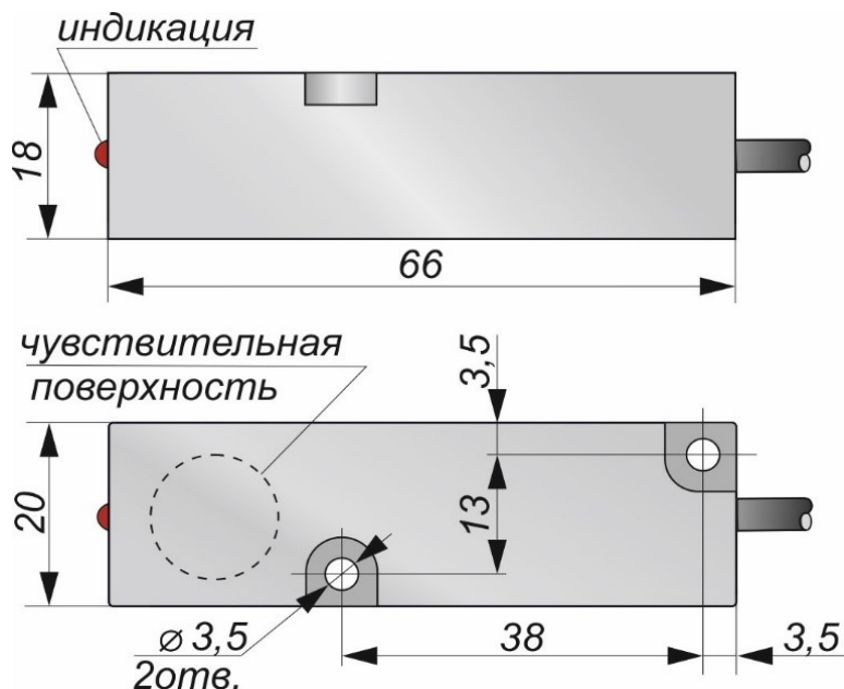
Габаритный чертеж
