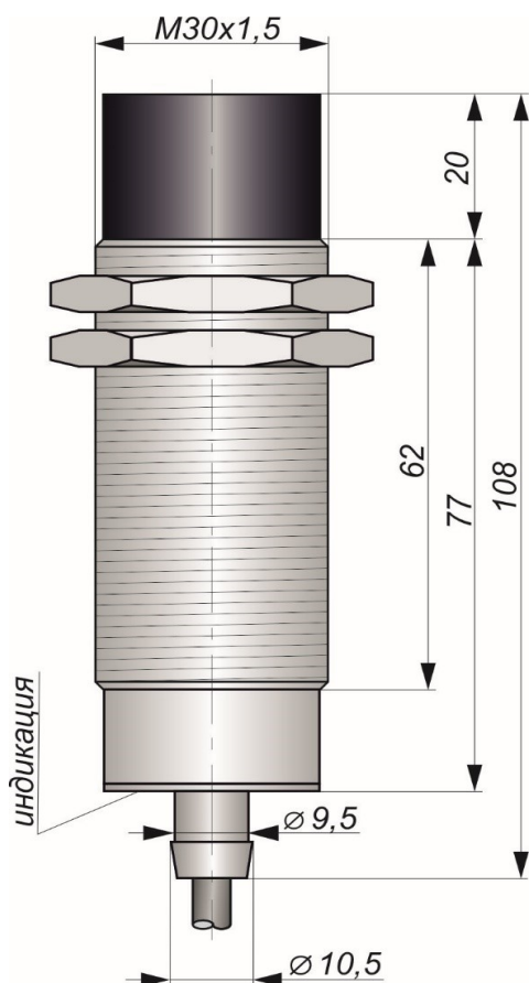
Габаритный чертеж
