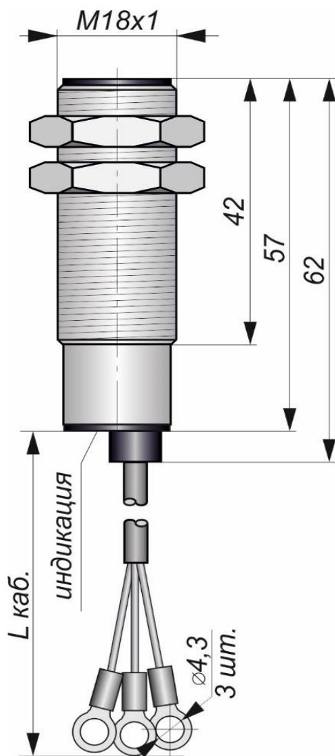
Габаритный чертеж
