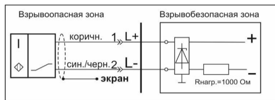
Схема соединения
