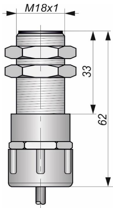
Габаритный чертеж
