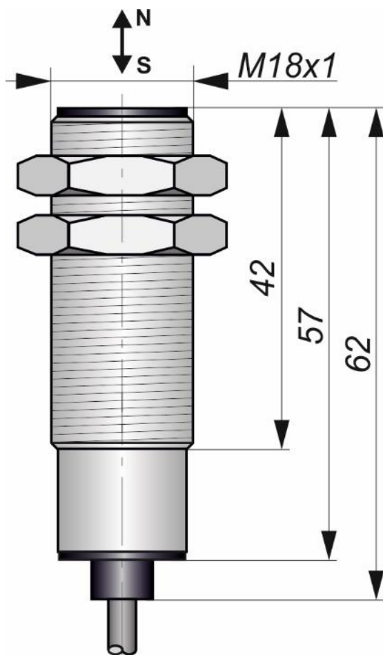
Габаритный чертеж
