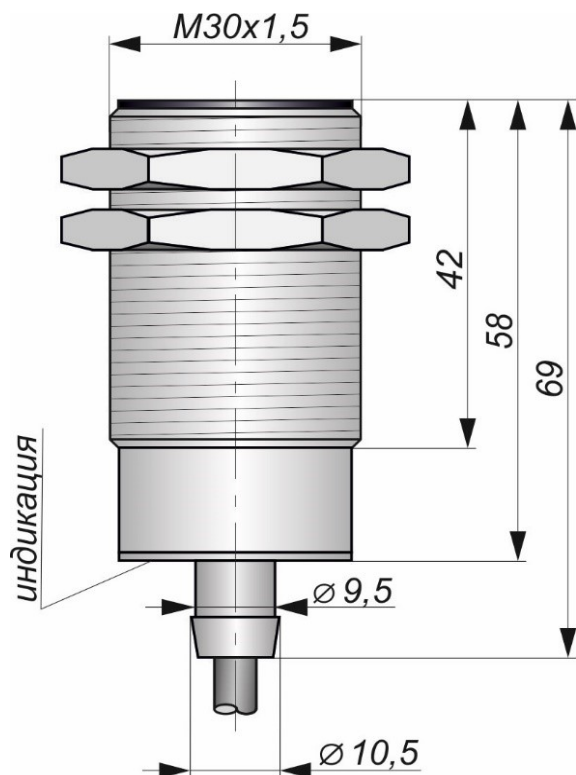
Габаритный чертеж
