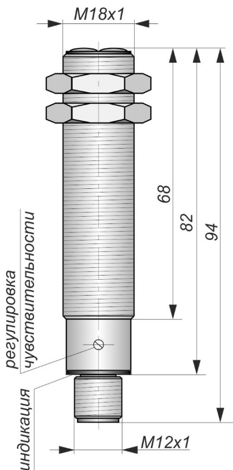
Габаритный чертеж
