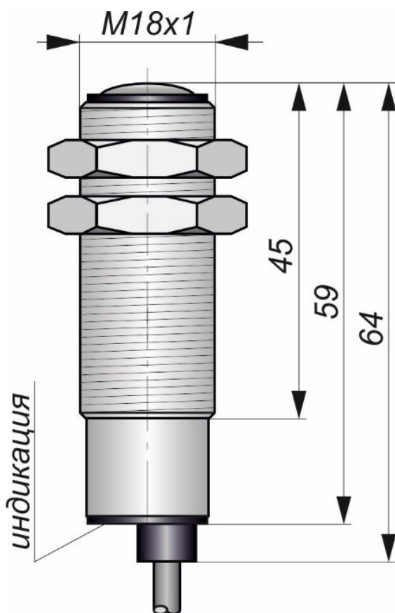
Габаритный чертеж
