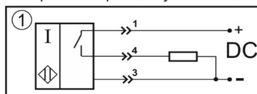
Схема соединения Нормально-разомкнутый контакт
