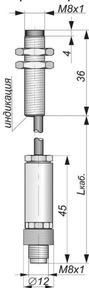
Габаритный чертеж
