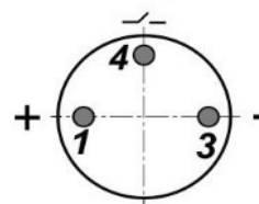
Цоколевка разъема
