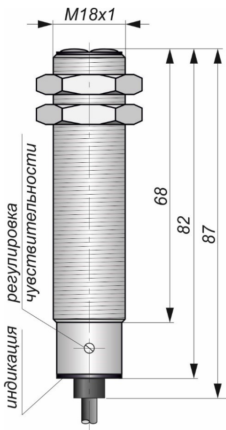
Габаритный чертеж
