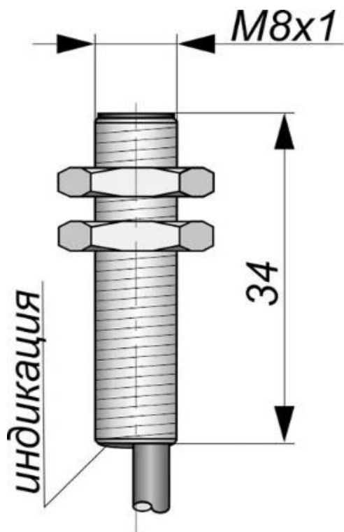
Габаритный чертеж
