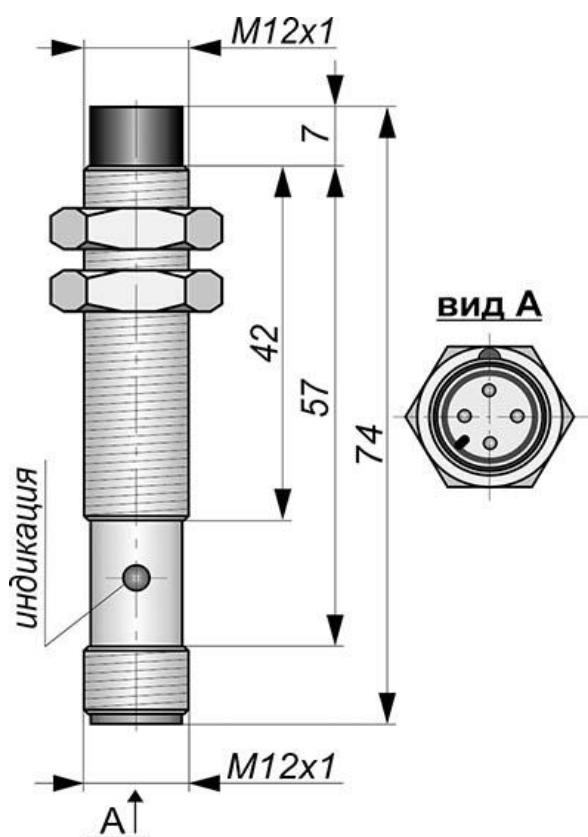
Габаритный чертеж
