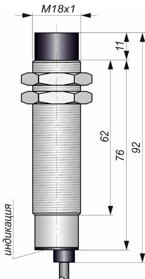
Габаритный чертеж
