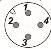
Цоколевка разъема
