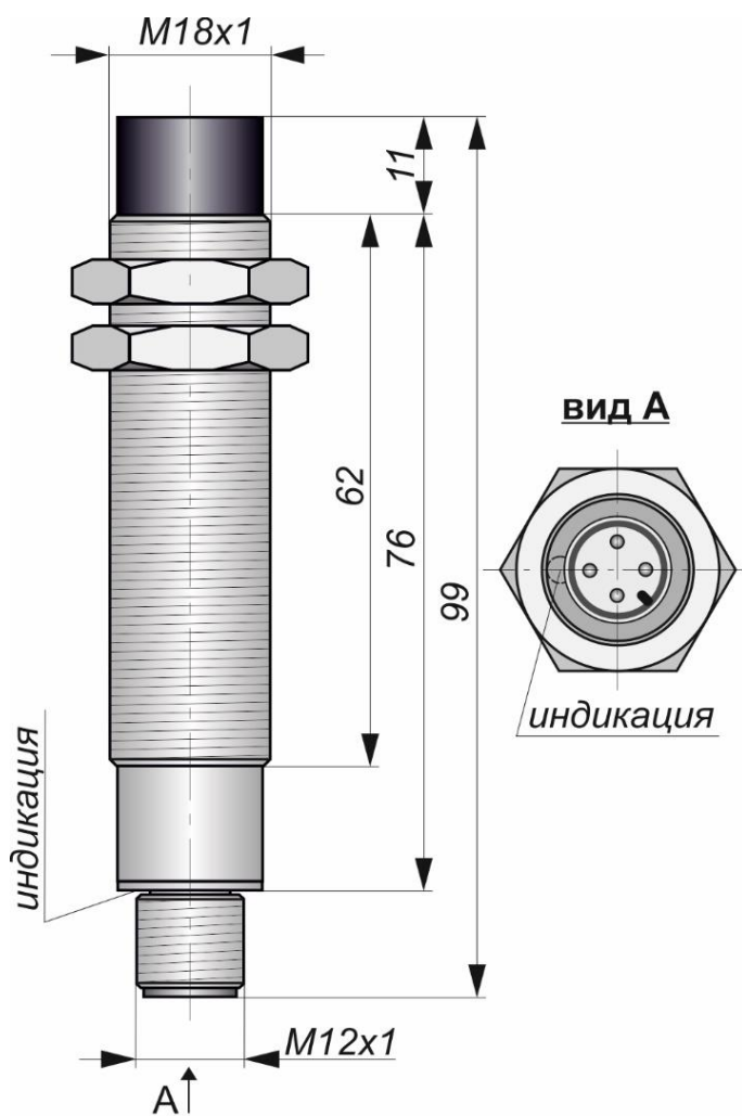
Габаритный чертеж
