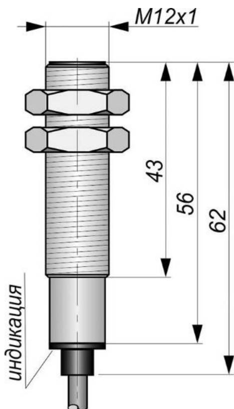
Габаритный чертеж
