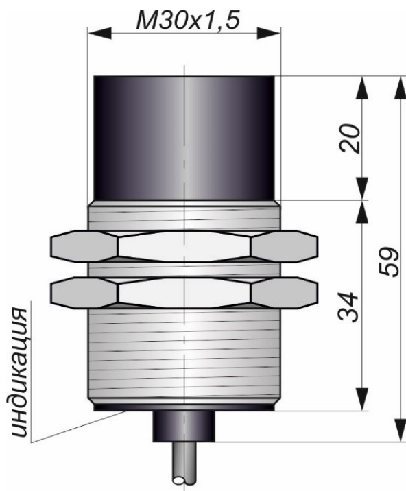
Габаритный чертеж
