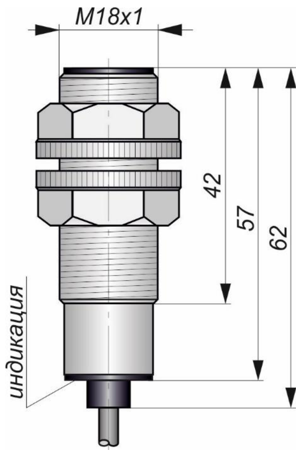
Габаритный чертеж
