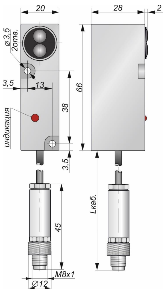
Габаритный чертеж
