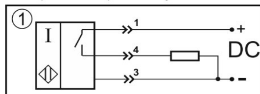
Цоколевка разъема
