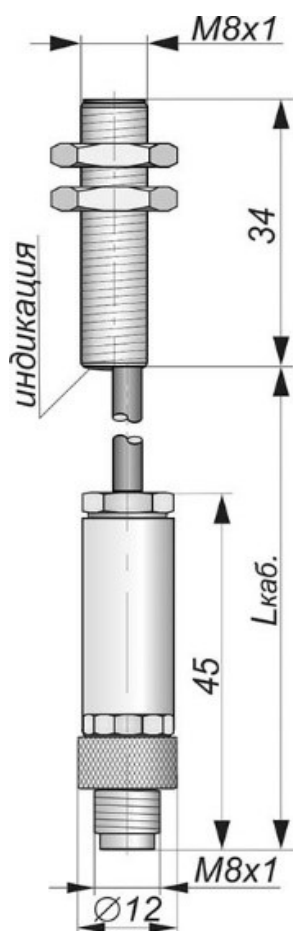
Габаритный чертеж
