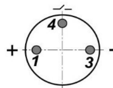
Цоколевка разъема
