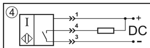
Цоколевка разъема
