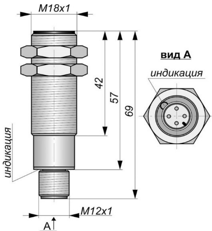
Габаритный чертеж
