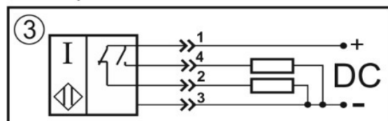
Переключающий контакт
