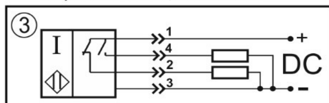
Переключающий контакт
