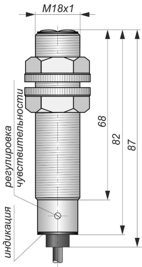
Габаритный чертеж
