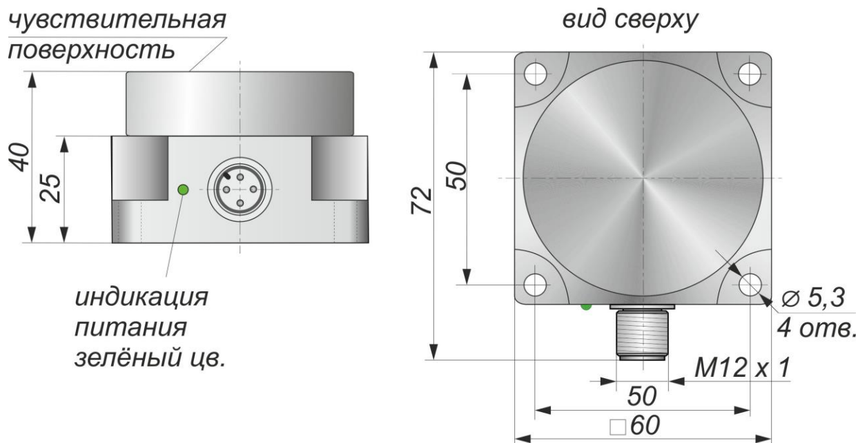
Габаритный чертеж
