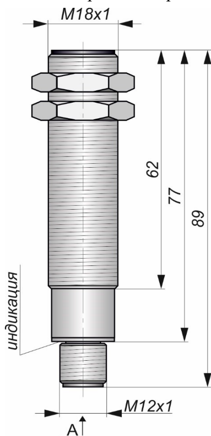
Габаритный чертеж
