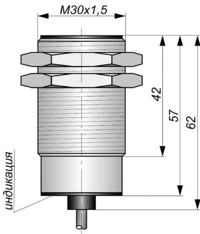
Габаритный чертеж
