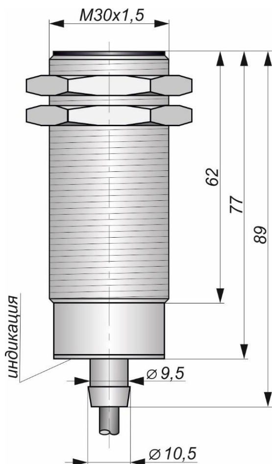
Габаритный чертеж
